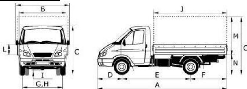
Габаритни размери:/мм/
